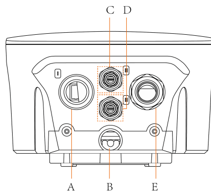
Abbildung 1-2 Anschlussdiagramm
