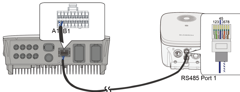
Abbildung 2-4 Mit Wechselrichter (SHRT) verbinden
