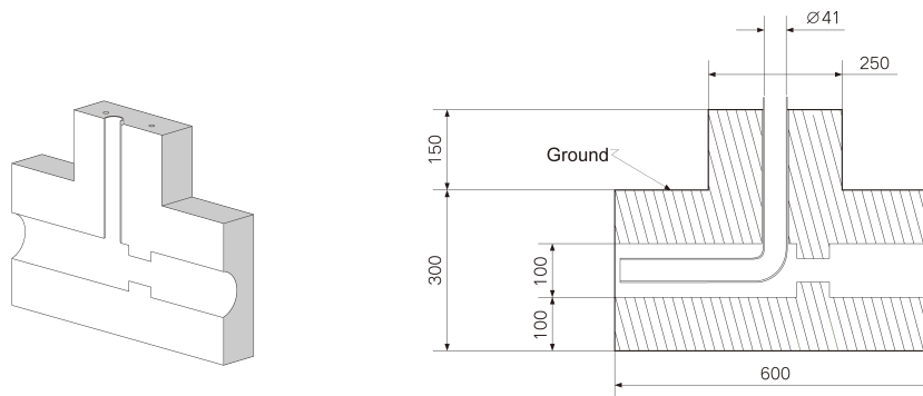
Abbildung 2-5 Vorderansicht (Einheit: mm)
