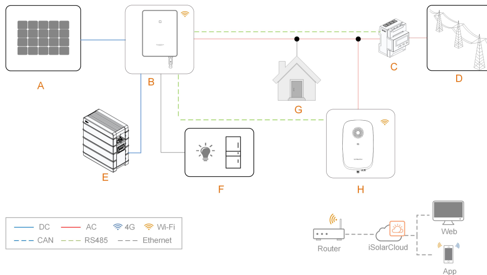
Abbildung 1-4 Systemtopologiediagramm der Lösung zum Laden und Speichern von Solarstrom
