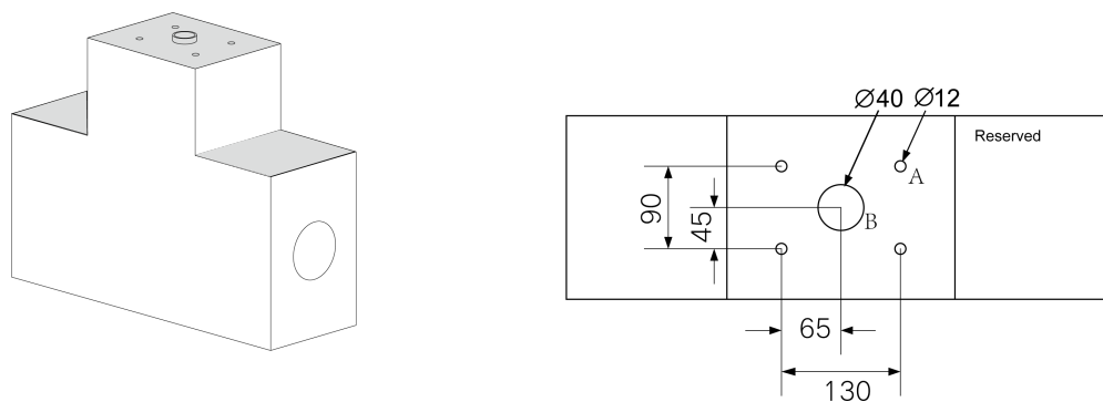
Abbildung 2-6 Draufsicht (Einheit: mm)
