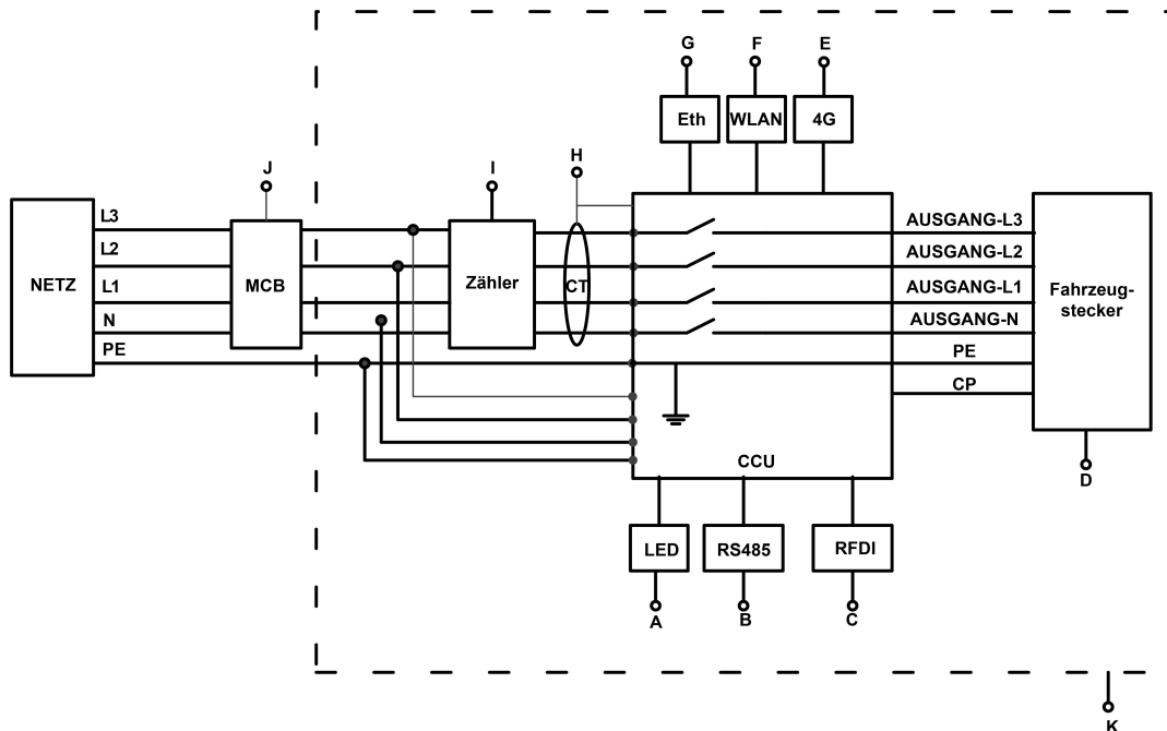
Abbildung 2-1 Schaltplan
