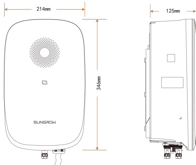
Abbildung 1-1 Erscheinungsbild und Abmessungen
