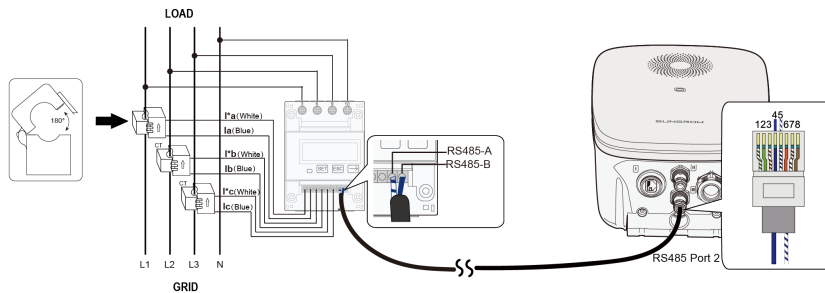
Abbildung 2-3 Mit Smart Energy Meter verbinden
